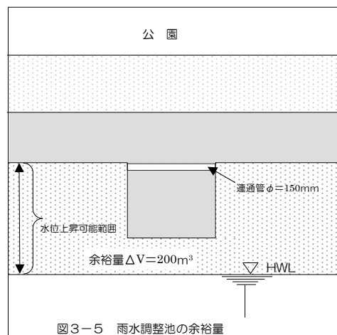
図 3-5 雨水調整池の余裕量
